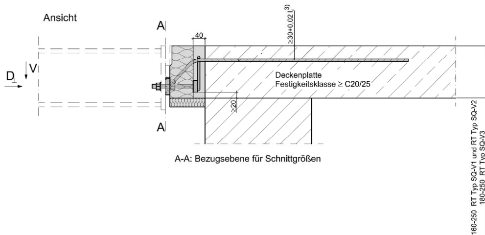
Abb. 18: Schöck Isokorb® RT Typ SQ-V1, Typ SQ-V2 und Typ SQ-V3, Schnittgrößendefinition
