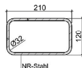
Abb. 8: Geschlossener Bügel 1 × Ø 8 mm
