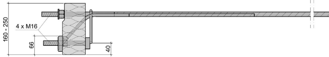
Abb. 24: Seitenansicht, Schöck Isokorb® RT Typ SK-M2
