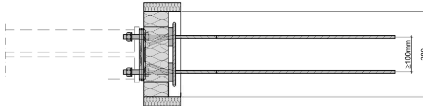
Abb. 11: Schöck Isokorb® RT Typ SQ-V1, Typ SQ-V2 und Typ SQ-V3, Grundriss
