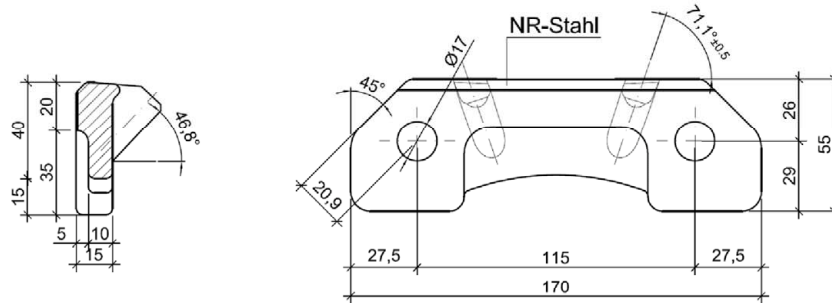
Abb. 9: Auflagerplatte
