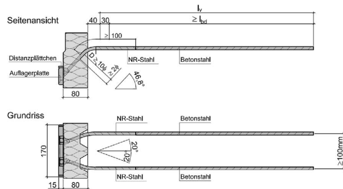
Abb. 13: Querkraftstäbe 2 × Ø inkl. Auflagerplatte
