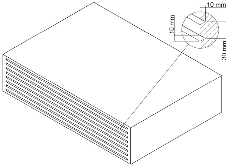
Abb. 28: Ausbildung einer rauhen Verbundfuge der Bestandsdecke
