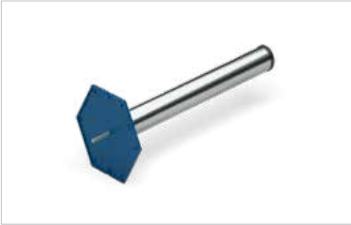
Schöck Stacon® type LD / F-LD Part S Gaine en acier inoxydable pour dilatation longitudinale. La platine plastique à clouer permet une fixation simple au coffrage
