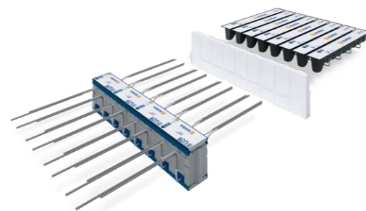
Schöck Isokorb® XT type K-ID
