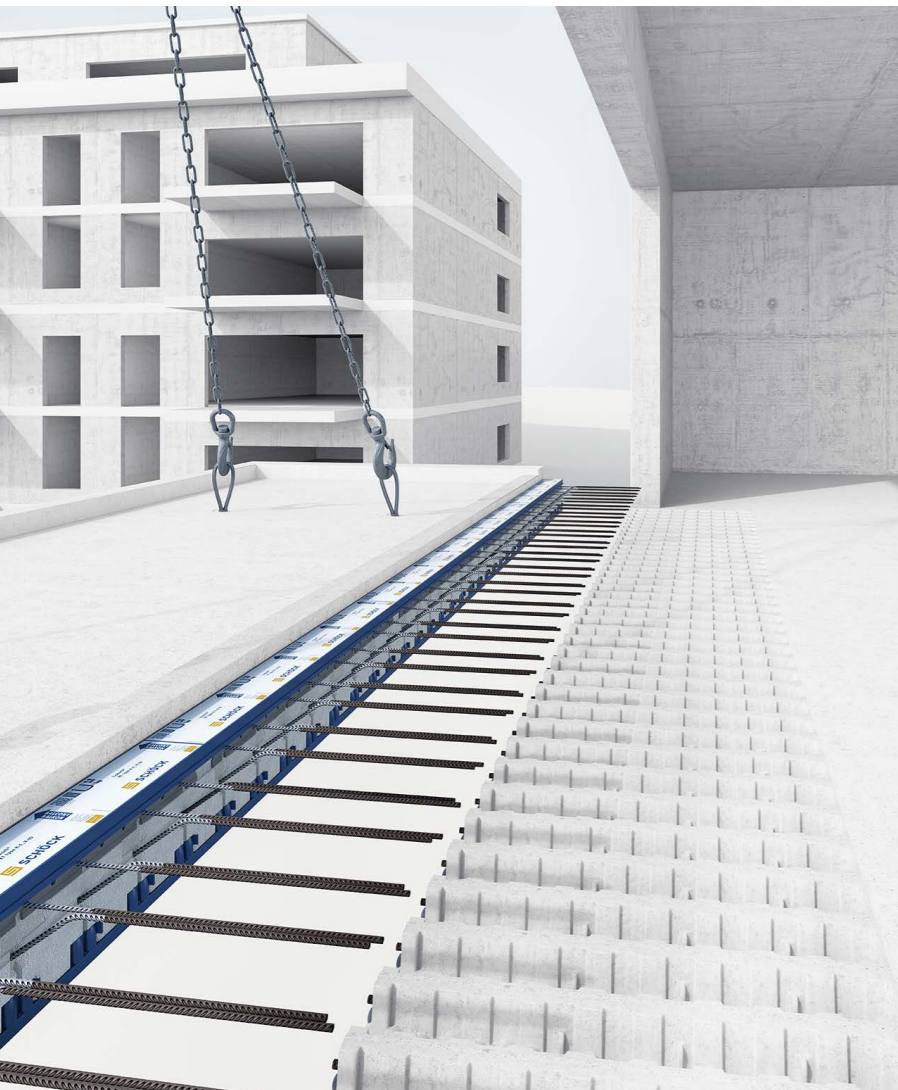
Schöck Isokorb® XT type K-ID
