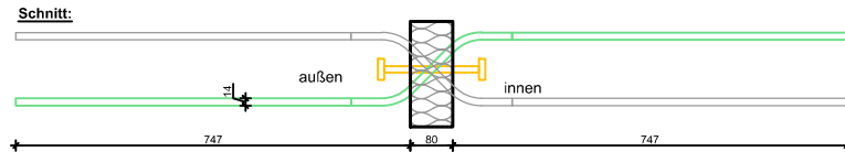
Schöck Isokorb T_D-MM2-VV2/3 bis T_D-MM5-VV2/3
