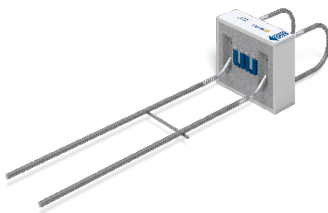
Schöck Isokorb T Typ Q Foto: Schöck Bauteile GmbH
