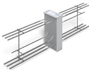
Schöck Isokorb T Typ B Foto: Schöck Bauteile GmbH
