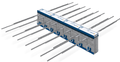
Schöck Isokorb T Typ K Foto: Schöck Bauteile GmbH
