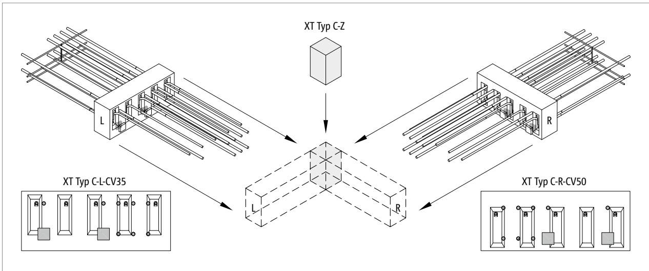
Abb. 217: Schöck Isokorb® XT Typ C-L-CV35, XT Typ C-R-CV50: Anordnung an der Ecke mit Eck-Dämmkörper
