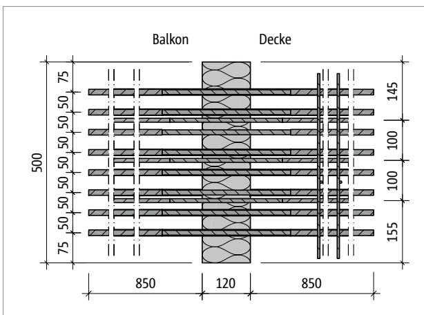
Abb. 45: Schöck Isokorb® XT Typ K-M13: Produktgrundriss
