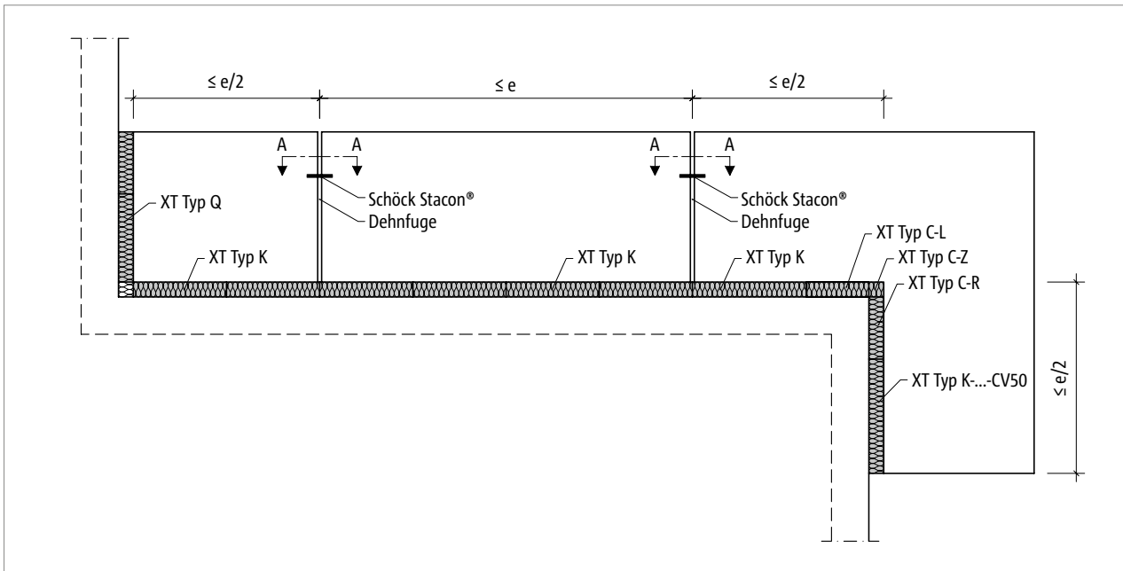
Abb. 16: Schöck Isokorb® XT Typ K: Dehnfugenausbildung mit längsverschieblichem Querkraftdorn, z. B. Schöck Stacon®
