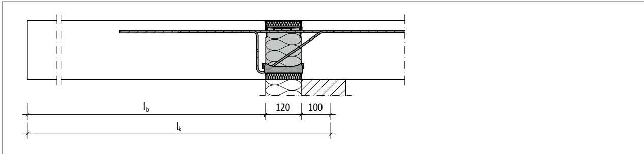
Abb. 10: Schöck Isokorb® XT Typ K: Systemkraglänge ( l_k ) für Bemessung und geometrische Kraglänge ( l_b )
