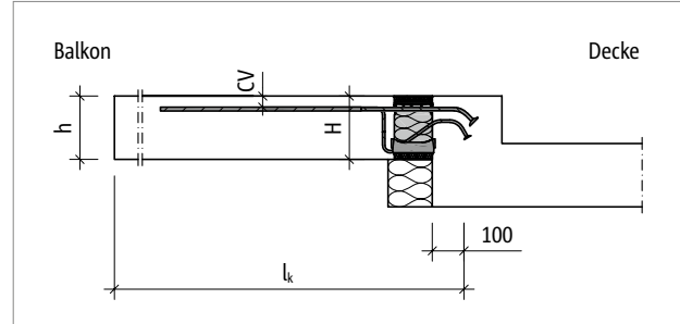
Abb. 97: Schöck Isokorb® XT Typ K-O: Statisches System
