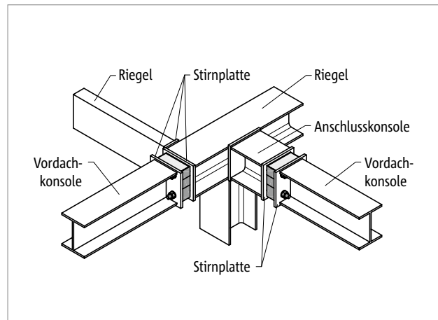
Abb. 236: Schöck Isokorb® T Typ S: Außenecke
