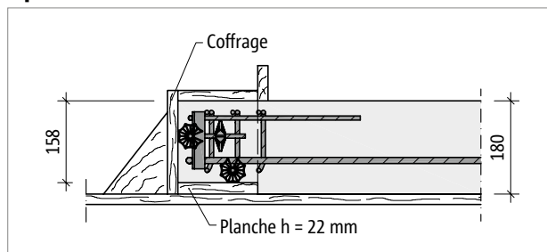
Ill. 45: Schöck Tronsole® type Z: réalisation d'une console d'appui sur le palier en préfabriqué, épaisseur de dalle de palier h = 180 mm
