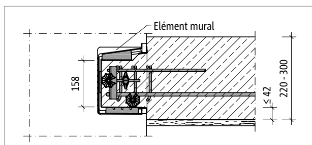
Ill. 43: Schöck Tronsole® type Z: élément mural sous forme de coffrage perdu, la cote inférieure du palier est plus basse que le cadre de raccordement de l'élément mural.
