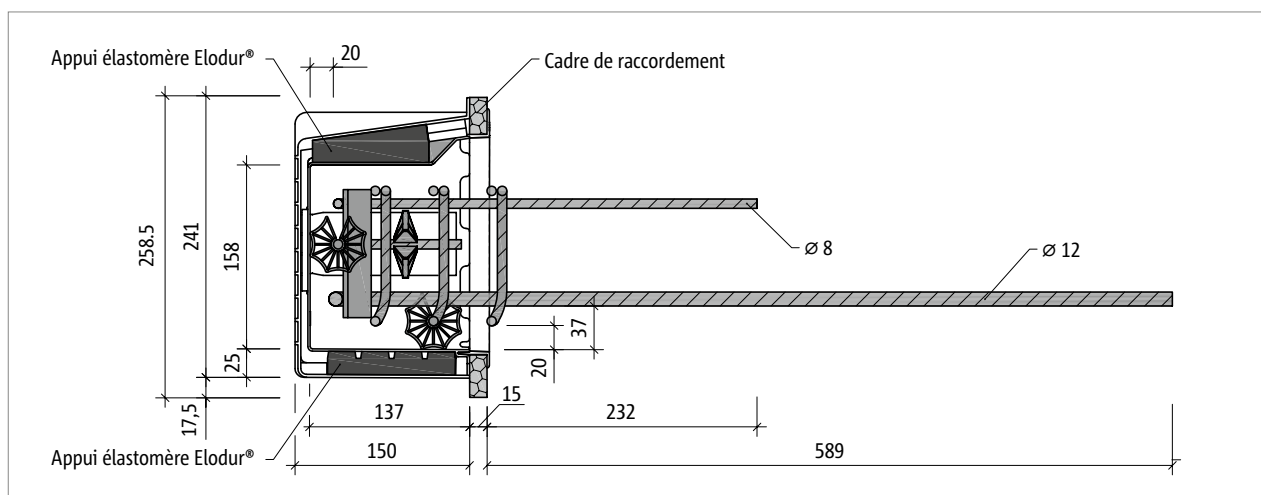
Ill. 54: Schöck Tronsole® type Z-V+V-T ou type Z-VH+VH-T: coupe verticale
