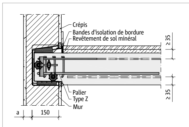
Ill. 61: Schöck Tronsole® type Z : Modèle de protection incendie
