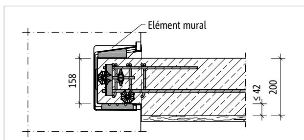
Ill. 42: Schöck Tronsole® type Z: élément mural sous forme de coffrage perdu, la cote inférieure du palier est plus basse que le cadre de raccordement de l'élément mural.
