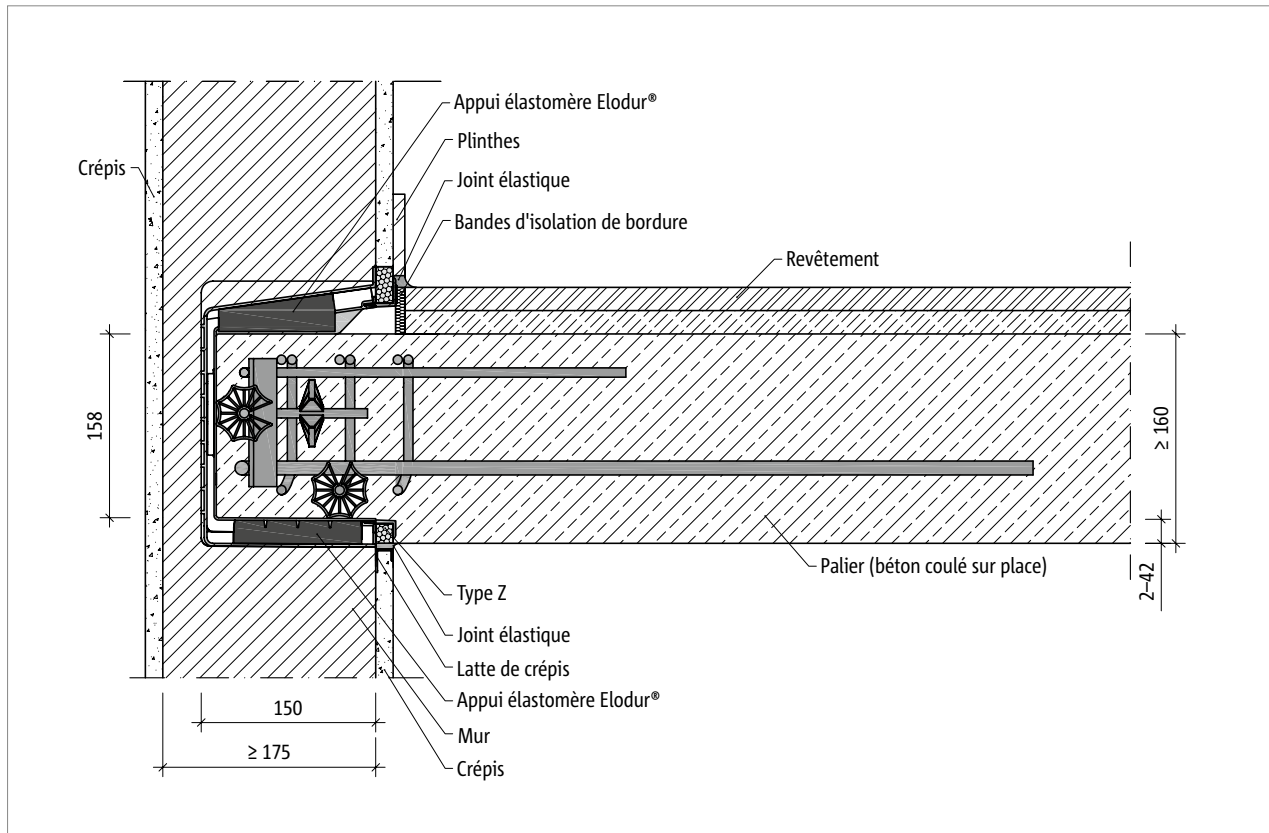
Ill. 48: Tronsole® Schöck type Z-V+V-T : coupe de montage palier en béton coulé sur place
