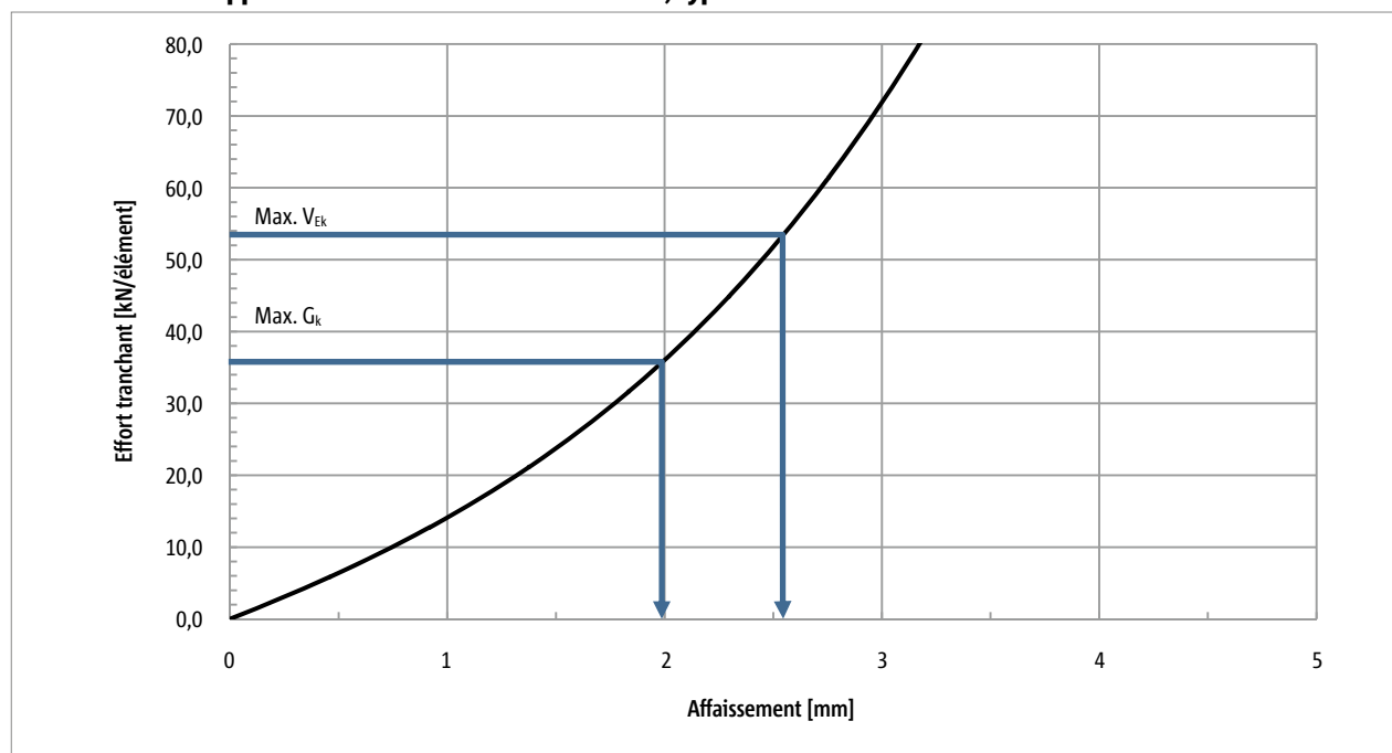
Ill. 59: Schöck Tronsole® type Z : Déformation de la couche élastomère Elodur®
