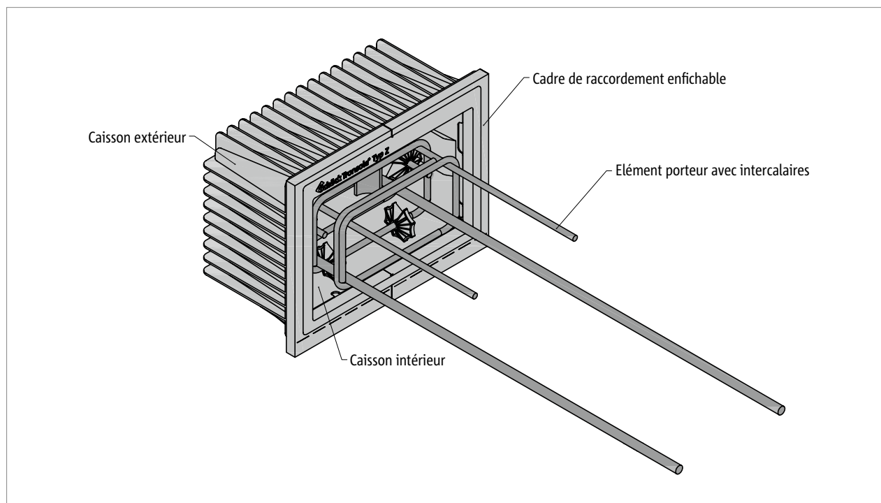
Ill. 39: Schöck Tronsole® type Z : élément mural composé d'un caisson extérieur, d'un caisson intérieur, d'un cadre de raccordement et de couches élastomère Elodur® intégrées (non visibles sur l'image). L'armature porteuse est disponible en option et est bétonnée dans le palier de l'escalier.
