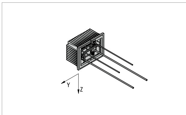
Ill. 57: Schöck Tronsole® type Z : convention de signes destinées au dimensionnement
