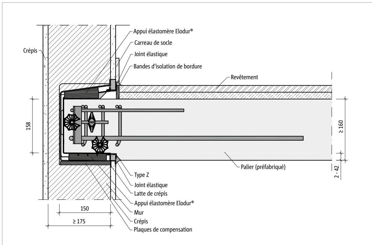
Ill. 49: Tronsole® Schöck type Z-V+V-T : coupe de montage palier en élément préfabriqué
