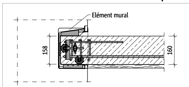
Ill. 40: Schöck Tronsole® type Z: élément mural comme coffrage perdu
