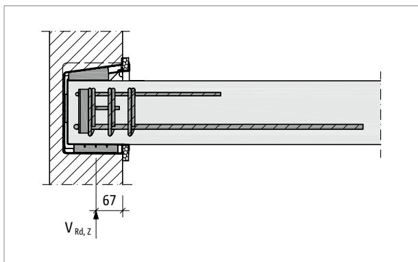
Ill. 58: Schöck Tronsole® type Z : représentation de la ligne d'impact de la force d'appui dans le mur
