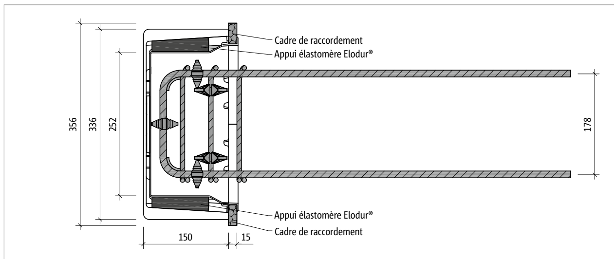
Ill. 53: Schöck Tronsole® type Z-VH+VH: coupe horizontale
