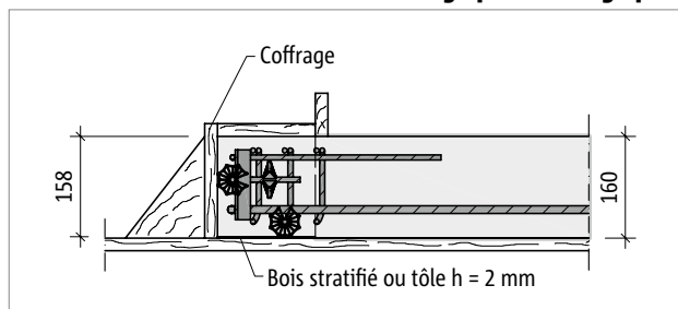
Ill. 44: Schöck Tronsole® type Z: réalisation d'une console d'appui sur le palier en préfabriqué, épaisseur de dalle de palier h = 160 mm
