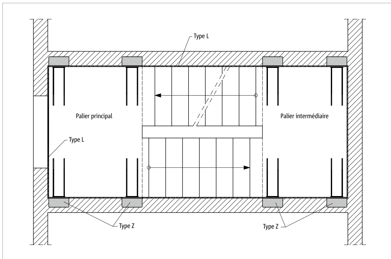
Ill. 50: Schöck Tronsole® type Z: disposition des éléments en plan
