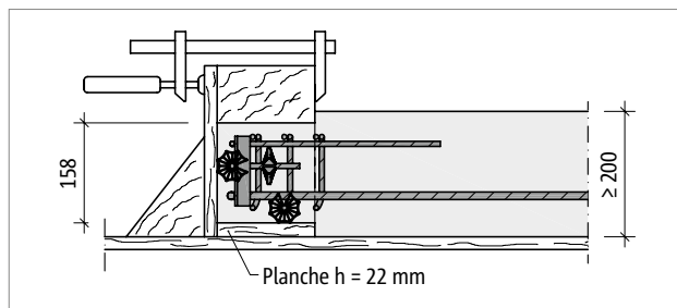
Ill. 46: Schöck Tronsole® type Z: réalisation d'une console d'appui sur le palier en éléments préfabriqués, épaisseur de dalle de palier h \geq 200 mm
