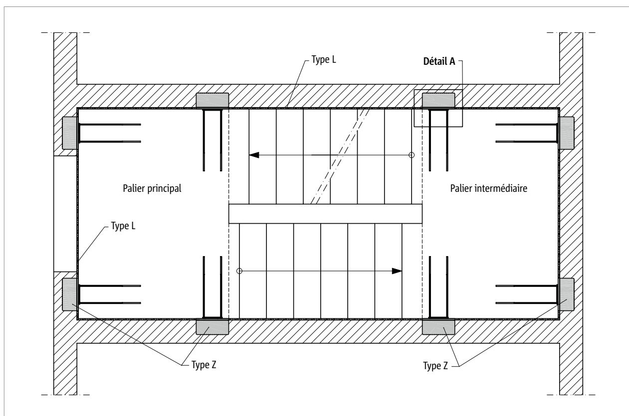
Ill. 51: Schöck Tronsole® type Z: alternative de la disposition des éléments en plan
