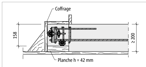
Ill. 47: Schöck Tronsole® type Z: réalisation d'une console d'appui sur le palier en éléments préfabriqués avec une différence de hauteur maximale entre les arêtes inférieures du palier et la console; épaisseur de dalle de palier h \geq 200 mm
