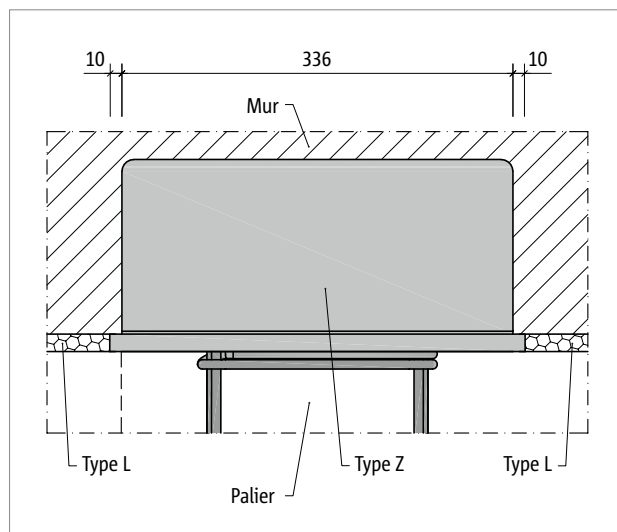
Ill. 52: Schöck Tronsole® type Z: disposition des éléments, détail A
