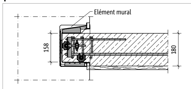
Ill. 41: Schöck Tronsole® type Z: élément mural comme coffrage perdu, la cote inférieure du palier est au même niveau que le cadre de raccordement de l'élément mural.
