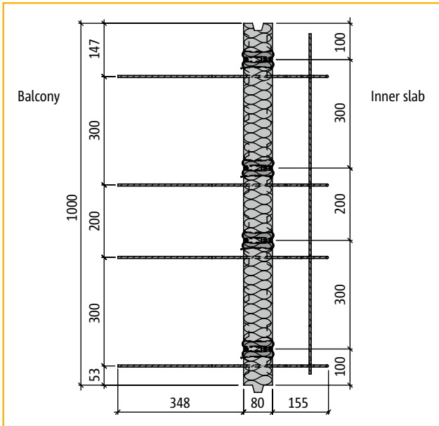
Plan view: Schöck Isokorb® type Q10
